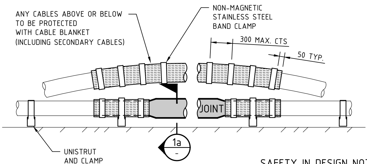
1 SECTION N.T.S
