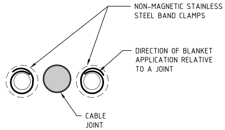
1a DETAIL N.T.S
